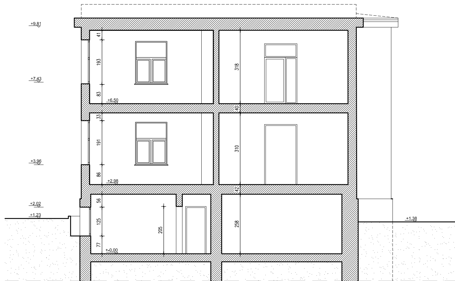
PRZEKRÓJ A-A
