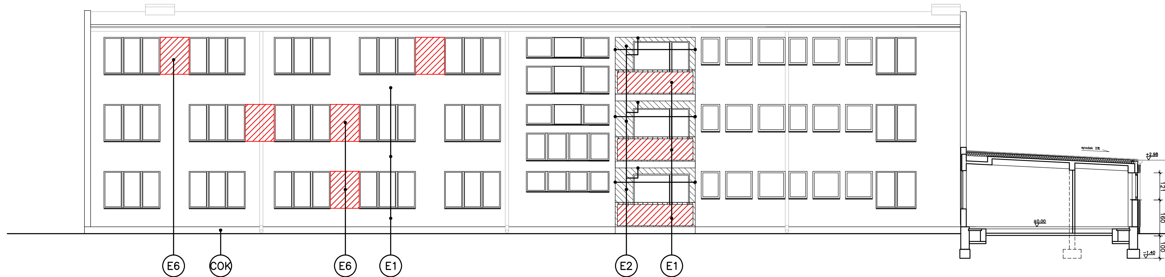
Budynek "D" EL. POŁUDNIOWA
