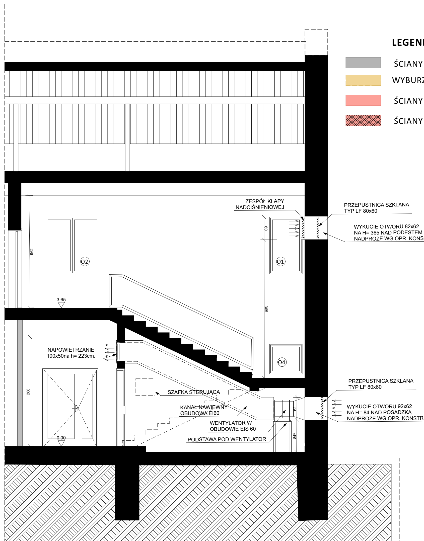
PRZEKRÓJ A1 -A1
