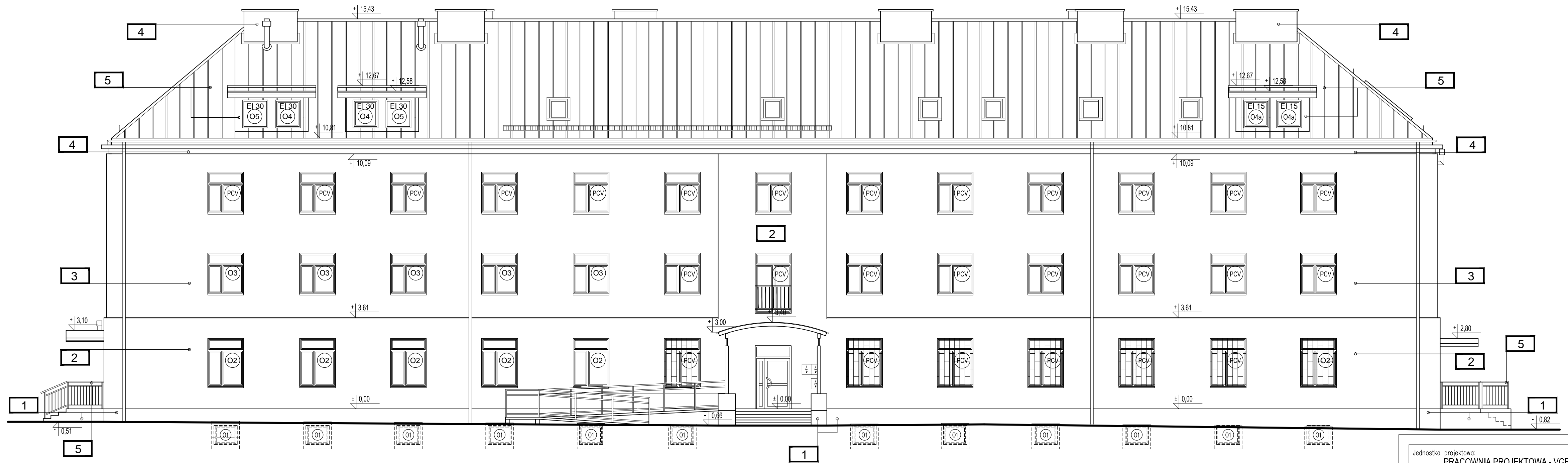
ELEWACJA ZACHODNIA
