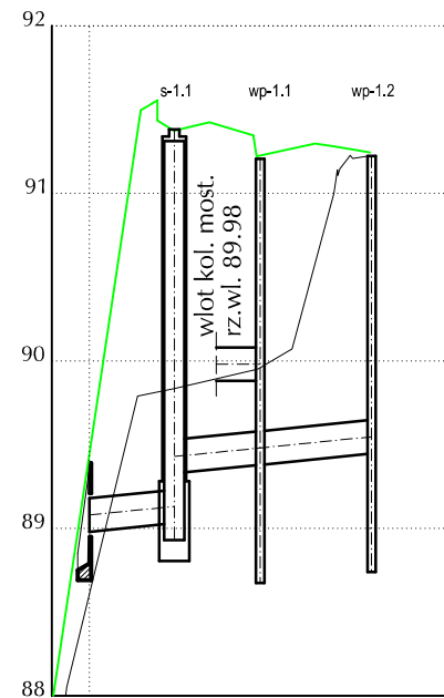
Kanalizacja KD-1
