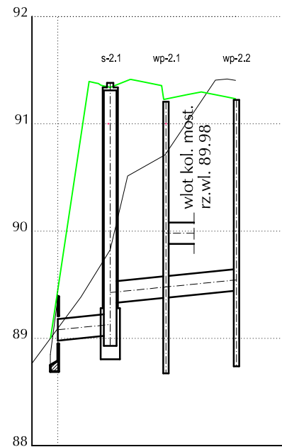
Kanalizacja KD-2
