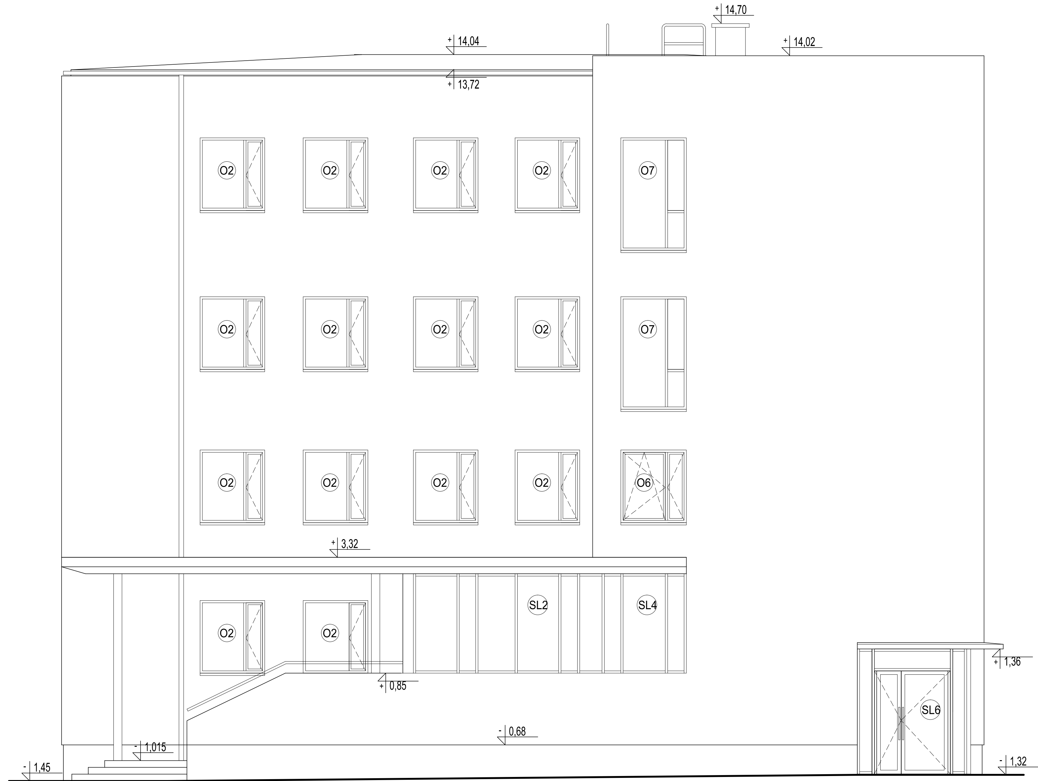
ELEWACJA PÓŁNOCNA
