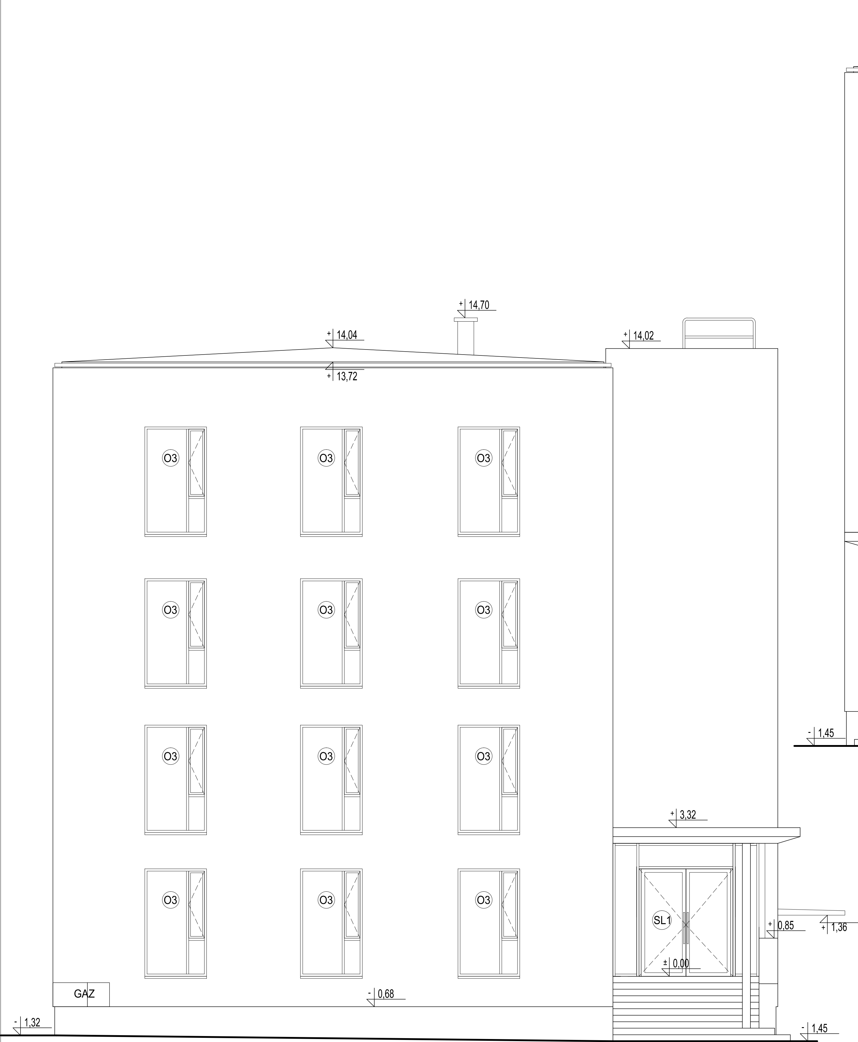
ELEWACJA WSCHODNIA
