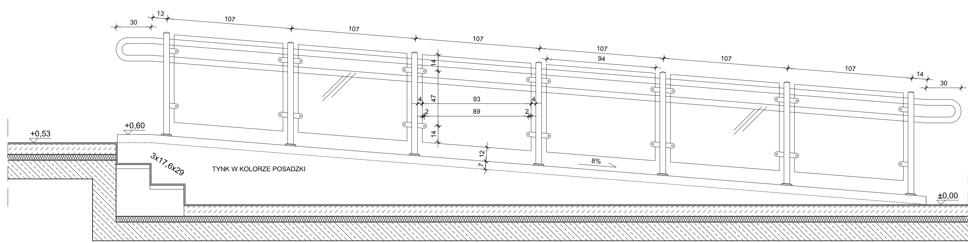
KONSTRUKCJA SCHODÓW I POCHYLNI WG PROJ. KONSTRUKCYJNEGO
