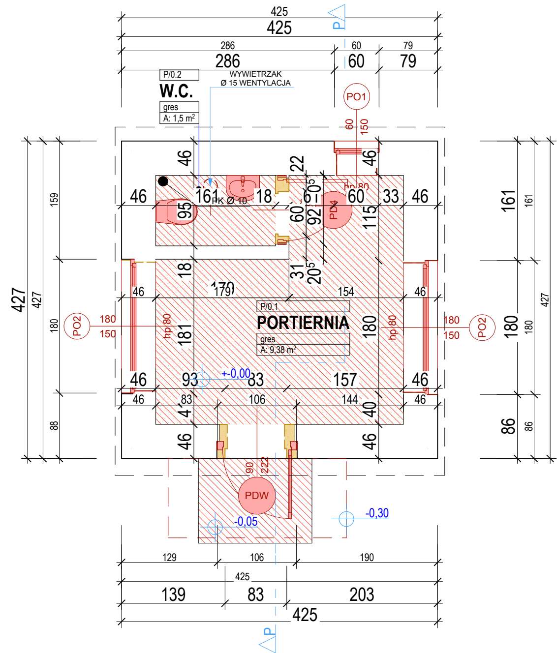
PROJEKT BUDOWLANY
