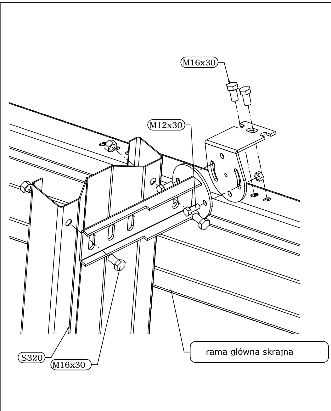
DETAL ŁĄCZNIKA SŁUPA SZCZYTOWEGO
