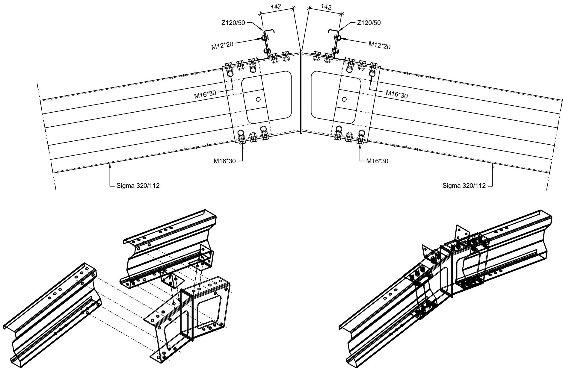
DETAL ŁĄCZNIKA KALENICOWEGO
