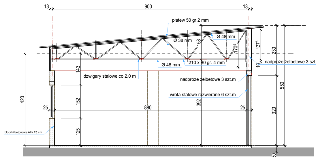
PRZEKRÓJ POPRZECZNY
