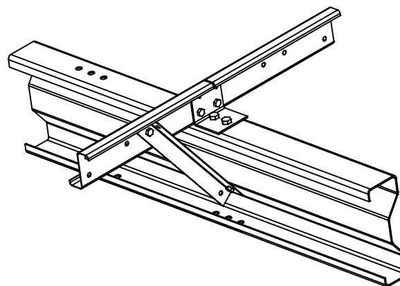
DETAL ZASTRZAŁU RYGLA DACHOWEGO
