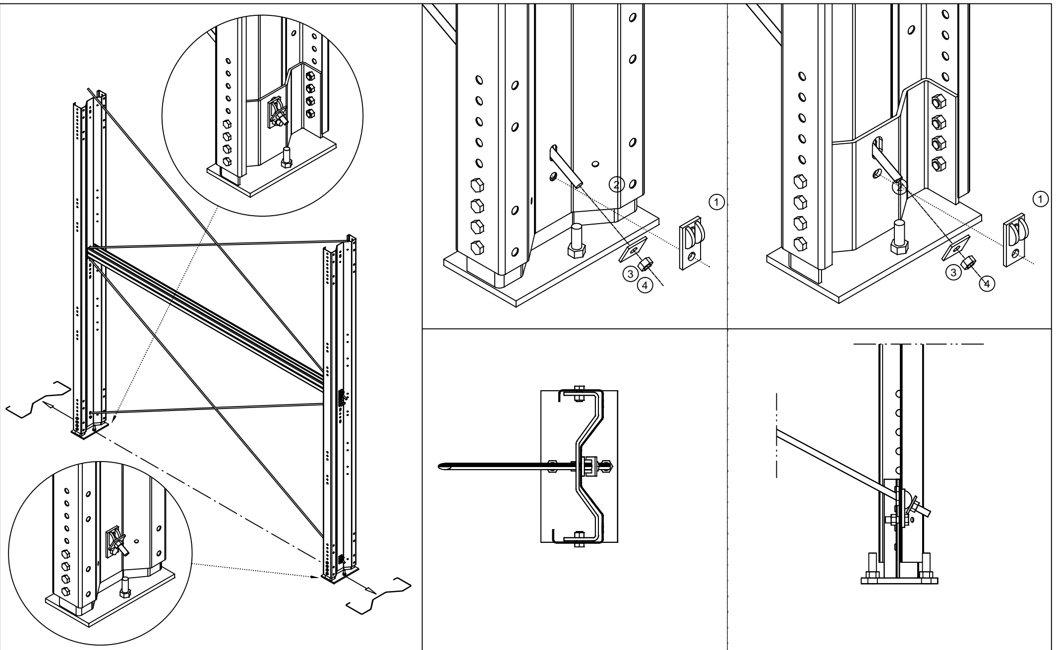
DETAL STĘŻENIA ŚCIAN - CZĘŚĆ DOLNA
