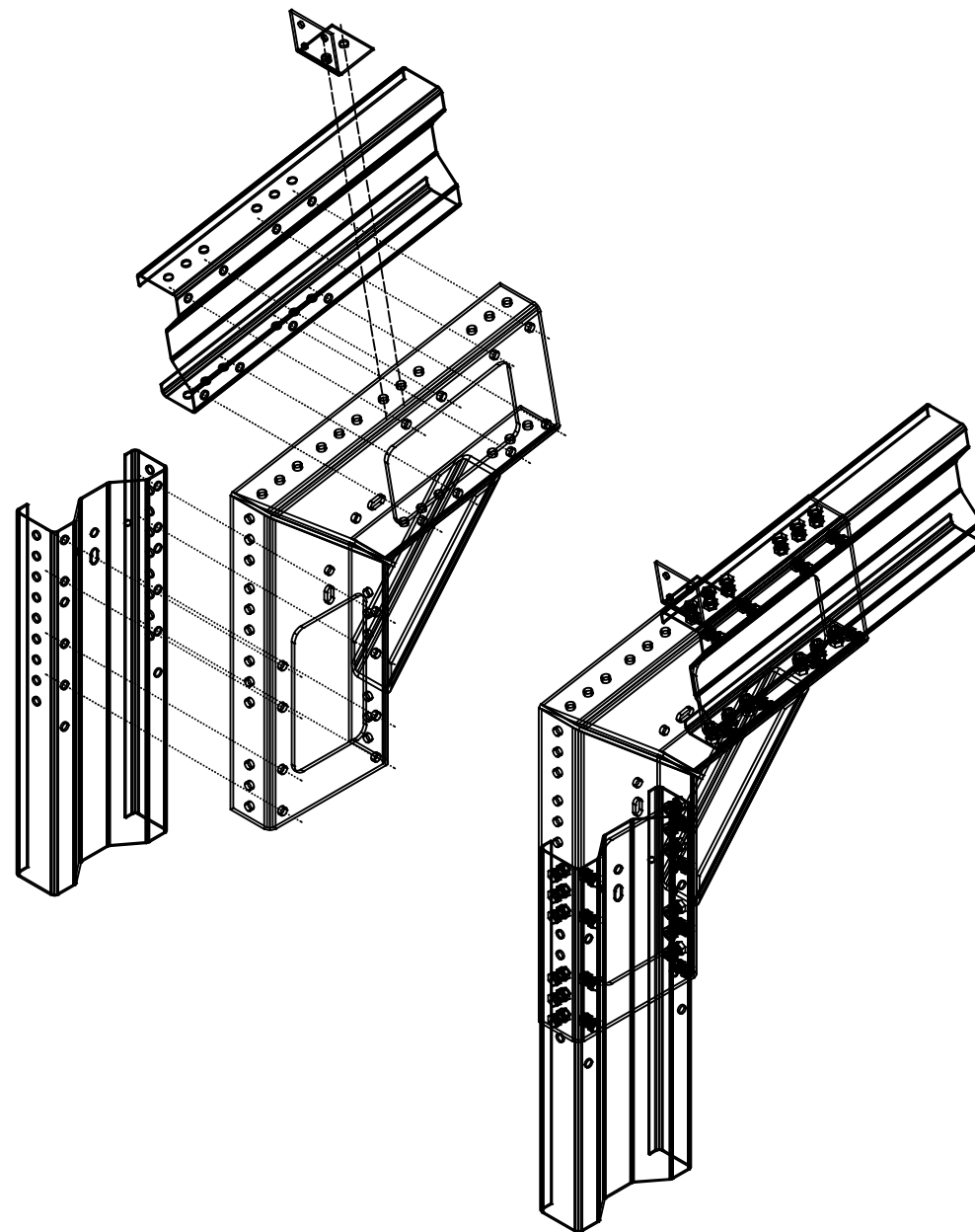
DETAL NAROŻA RAMY GŁÓWNEJ
