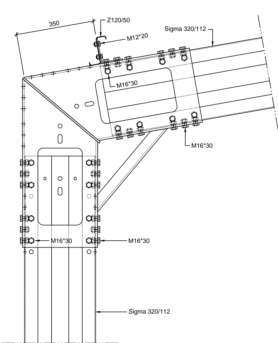
DETAL NAROŻA RAMY GŁÓWNEJ
