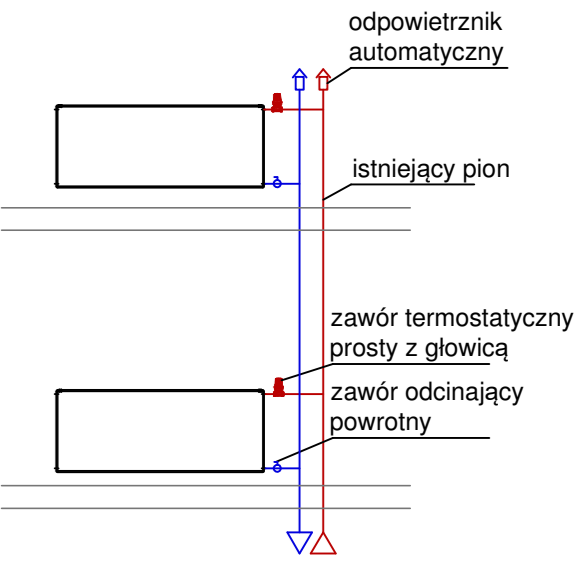
schemat montażowy
