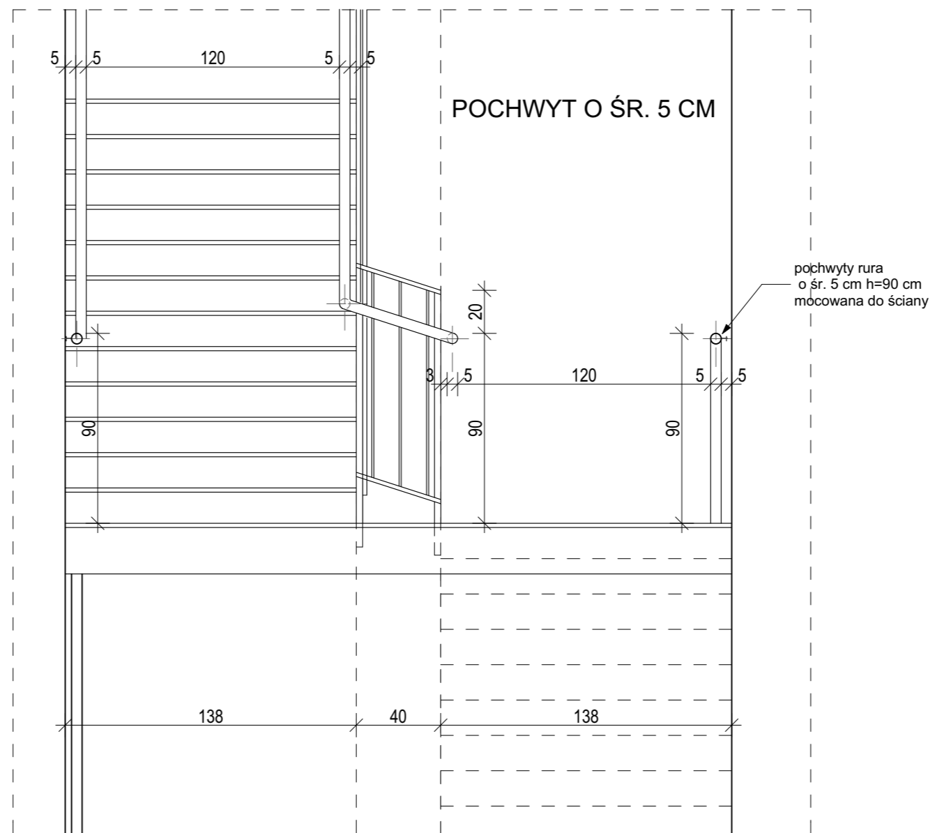
DETALE BARIER SCHODOWYCH 1:25
