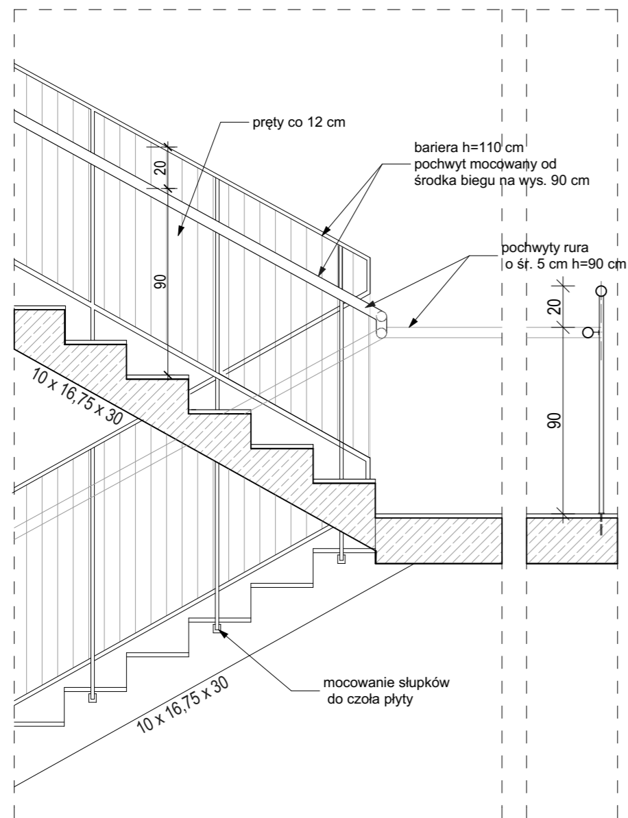
PORĘCZE ZE STALI MALOWANEJ PROSZKOWO NA KOLOR SZARY
