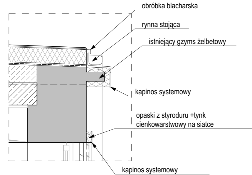
DETAL GZYMSU 1 : 20
