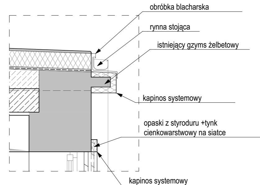
DETAL GZYMSU 1 : 20
