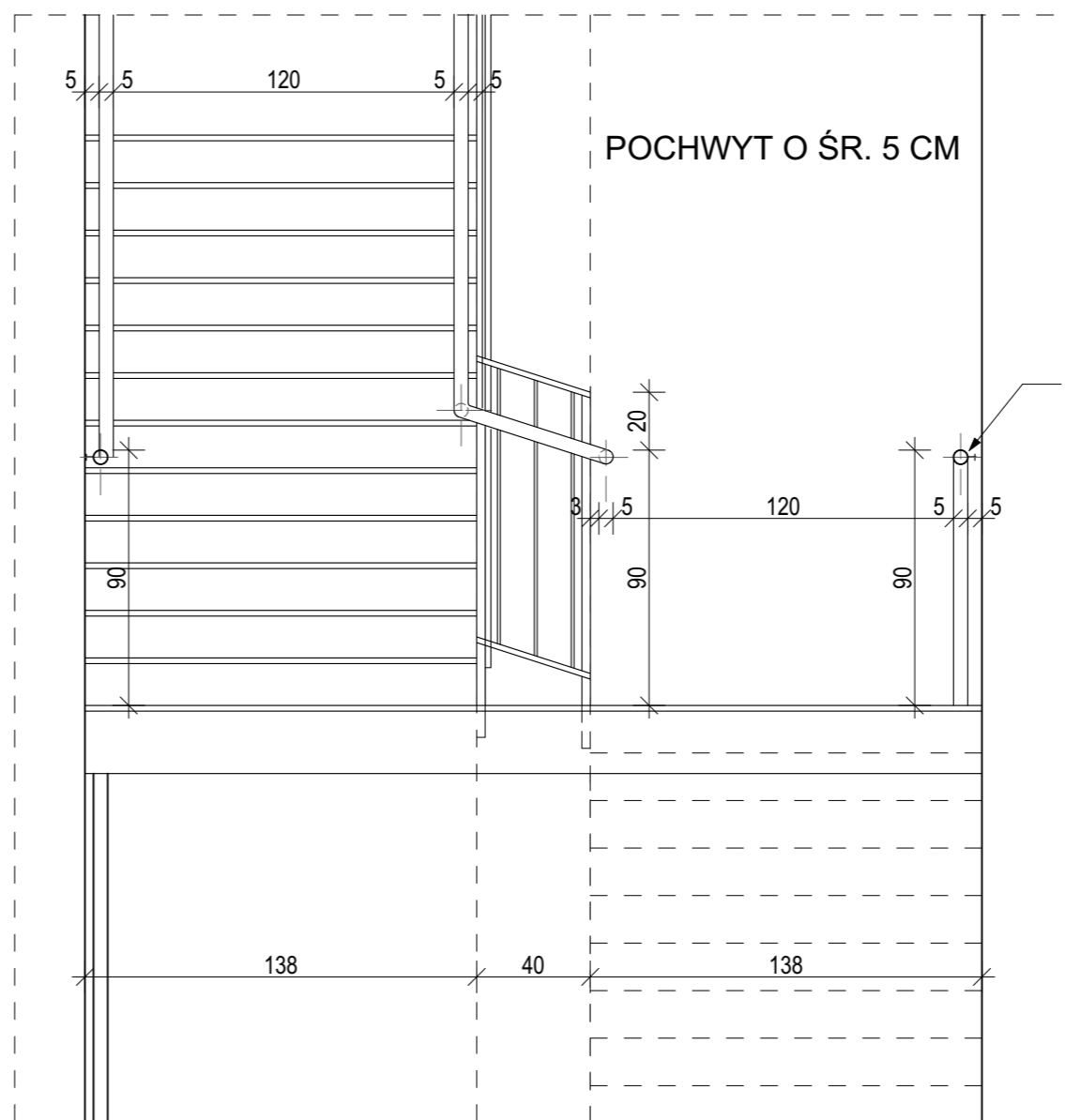
DETALE BARIER SCHODOWYCH 1:25
